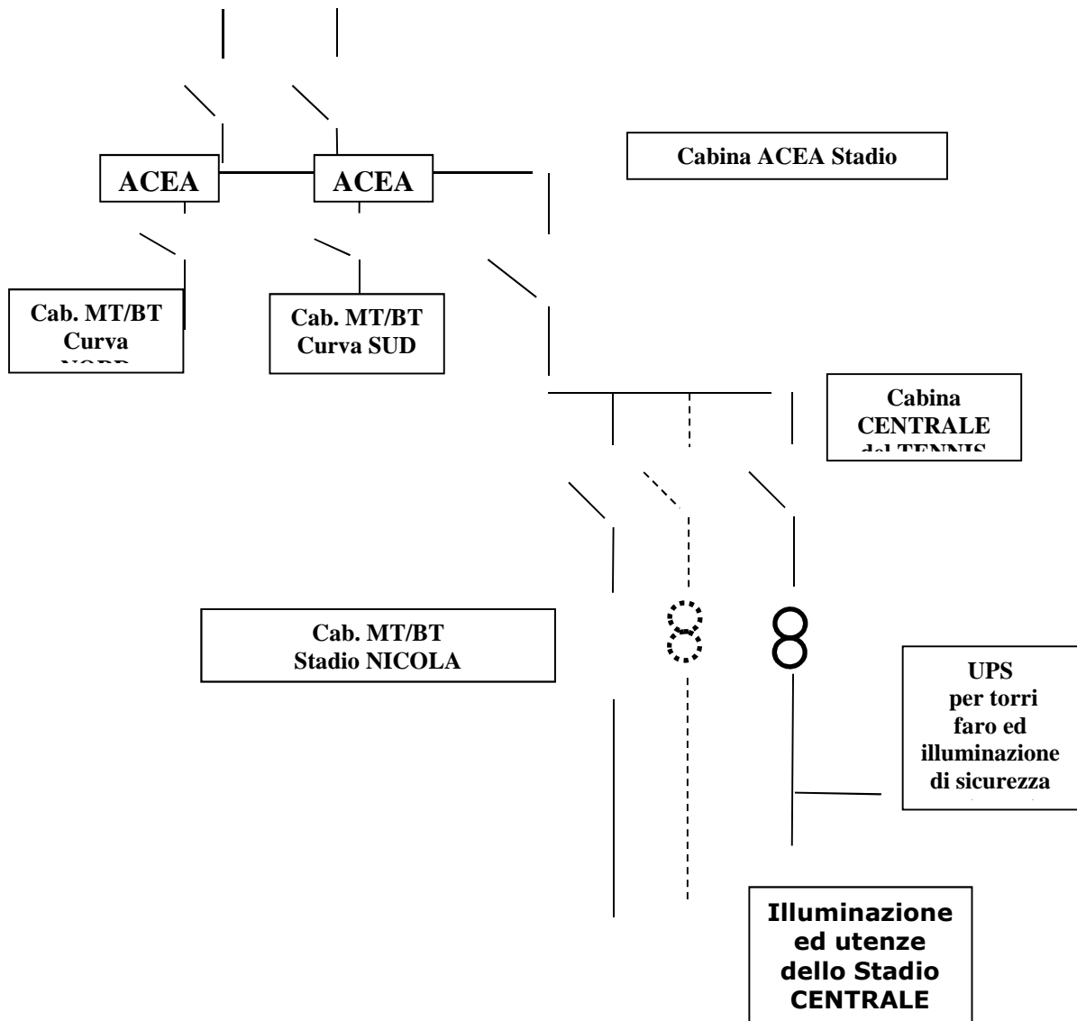
Fig. 11 – Schema a blocchi dell'impianto elettrico residente
